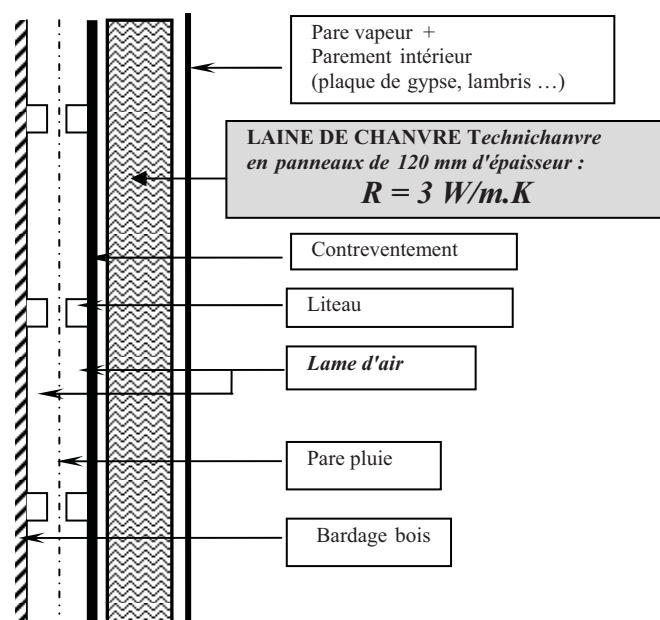
Coupe transversale d' UNE OSSATURE BOIS VERTICALE
