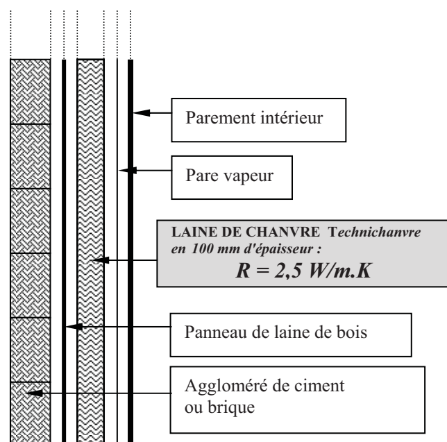
Coupe transversale d' UNE MAÇONNERIE EXTÉRIEURE
